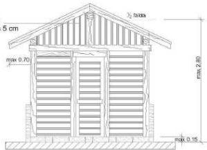
PROSPETTO FRONTALE
