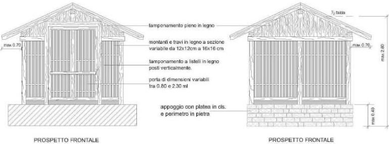
PROSPETTO FRONTALE
