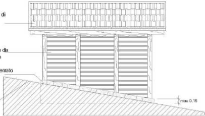
PROSPETTO LATERALE
