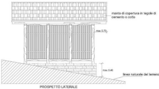
PROSPETTO LATERALE
